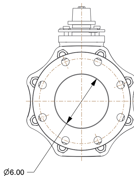
ISO 5211-F12
